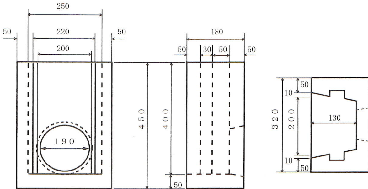
寸法図
