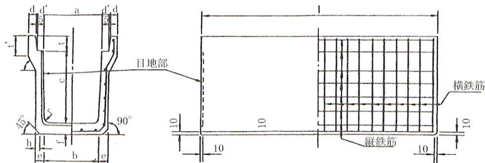
形状・寸法及び配筋
