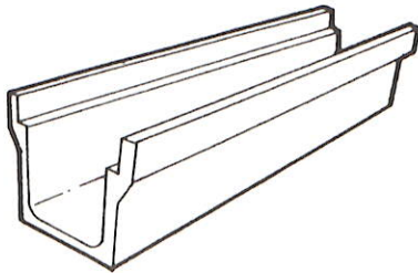
形状・寸法及び配筋
