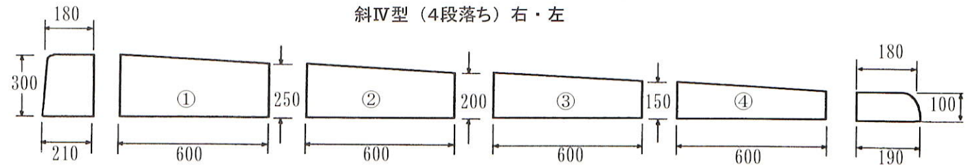
斜Ⅳ型（大阪府型4段落ち）右・左
