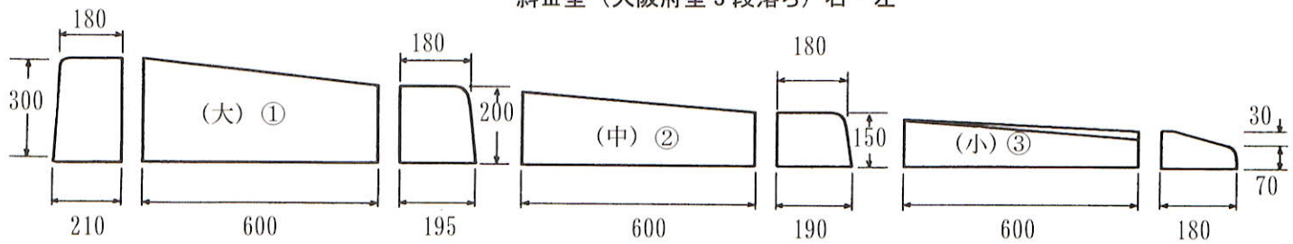
斜Ⅲ型（大阪府型3段落ち）右・左
