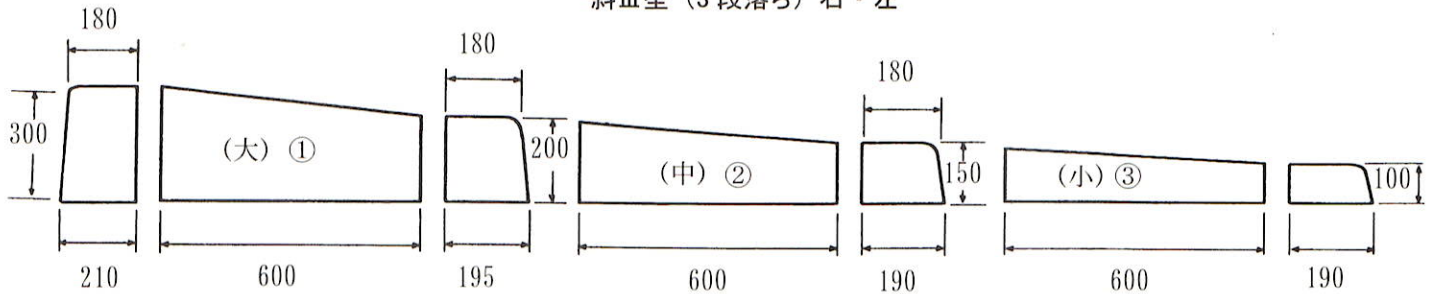
斜Ⅲ型（3段落ち）右・左
