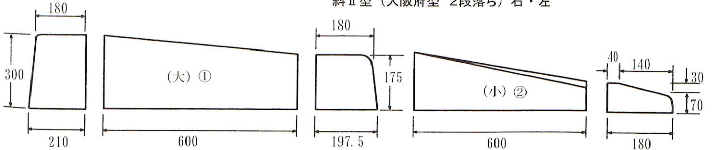
斜Ⅱ型（大阪府型 2段落ち）右・左
