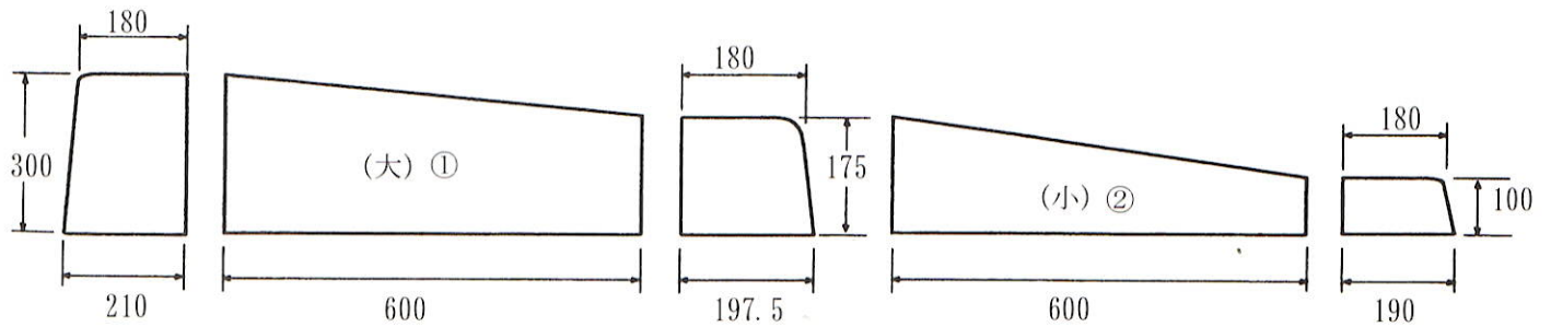
斜Ⅱ型（2段落ち）右・左
