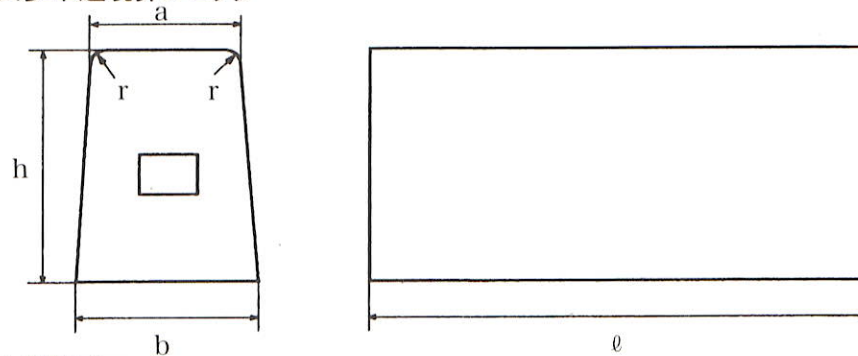
地先境界ブロック
