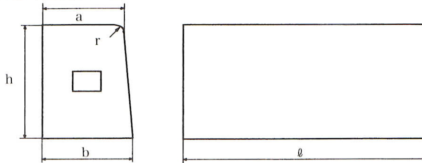
片面歩車道境界ブロック
