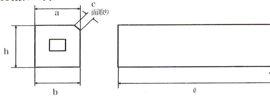
地先境界ブロック
