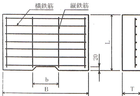
寸法・配筋・質量表
