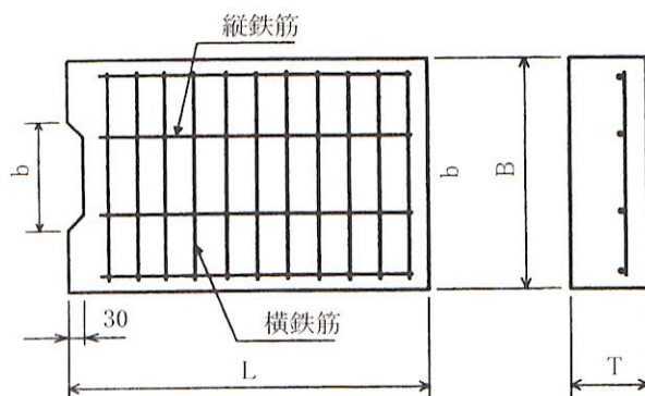
寸法・配筋・重量表
