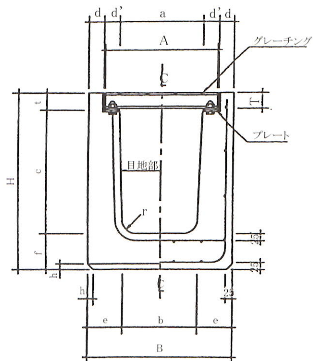
断面図
