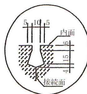
目地部詳細図
